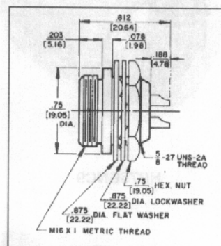
CB-3M
