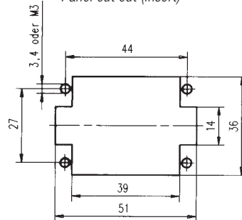
Montageausschnitt (Kontaktträger) Panel cut out (insert)
