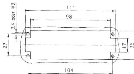
Montageausschnitt (Kontaktträger) Panel cut out (insert)
