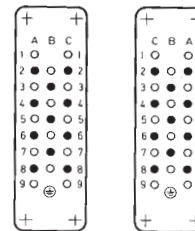
Buchseinsatz Female insert
