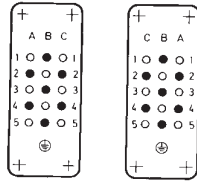
Buchseinsatz Female insert
