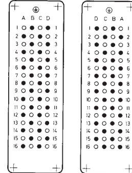
Buchseinsatz Female insert
