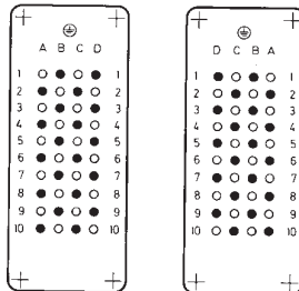
Buchseinsatz Female insert
