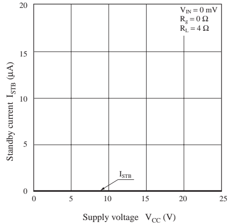
I_{STB} — V_{CC}
