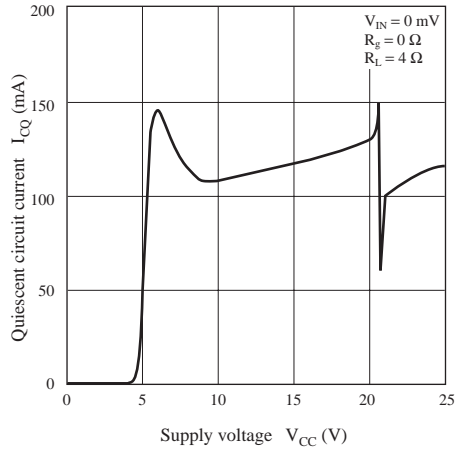
I_{CQ} — V_{CC}
