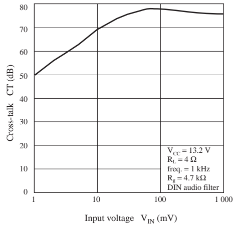
CT — V_{IN}
