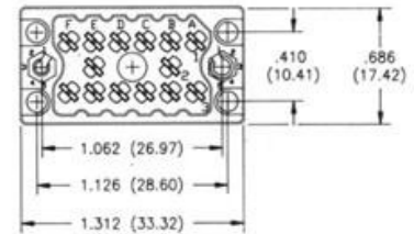
36 PIN RECEPTACLE
