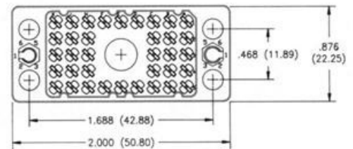
36 PIN RECEPTACLE
