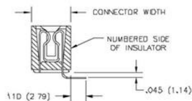
CONTACT CODE 553
