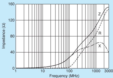
BLM03EB250SZ1
