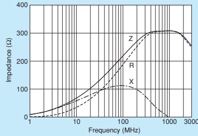
BLM18EG221TZ1/BLM18EG221TH1
