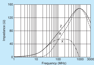
BLM15BX750SZ1
