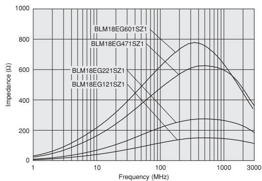
BLM18EG_SZ1 Series
