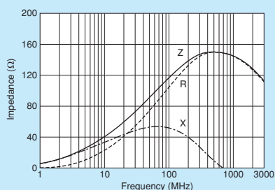
BLM18EG121SZ1/BLM18EG121SH1
