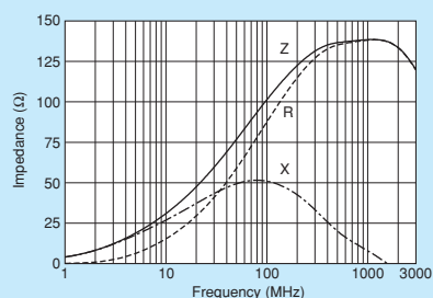
BLM18EG101TZ1/BLM18EG101TH1
