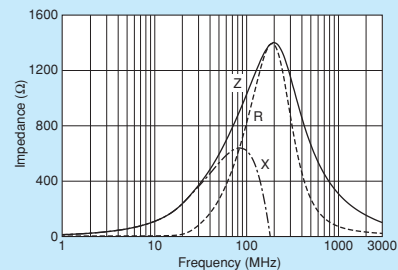
BLM15BX102SZ1
