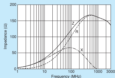
BLM15EG121SZ1
