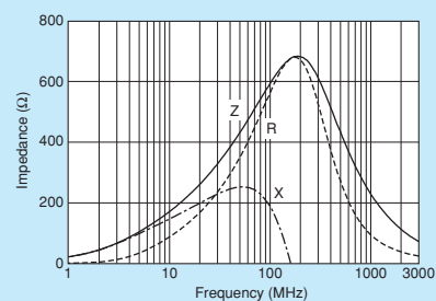
BLM18AG601SZ1/BLM18AG601SH1
