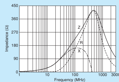
BLM15BX221SZ1
