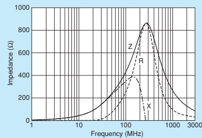
BLM18BD421SZ1/BLM18BD421SH1
