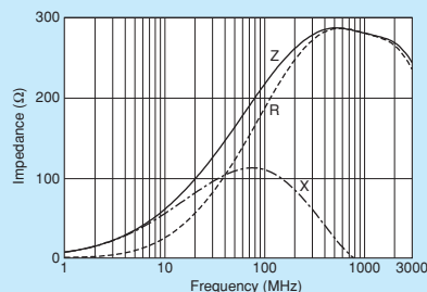
BLM15EG221SZ1
