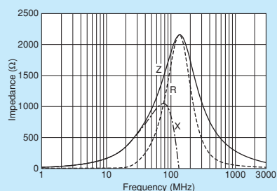
BLM15BX182SZ1
