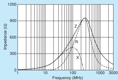
BLM15BX601SZ1
