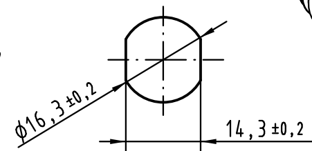
Montageausschnitt panel cut out (1:1)
