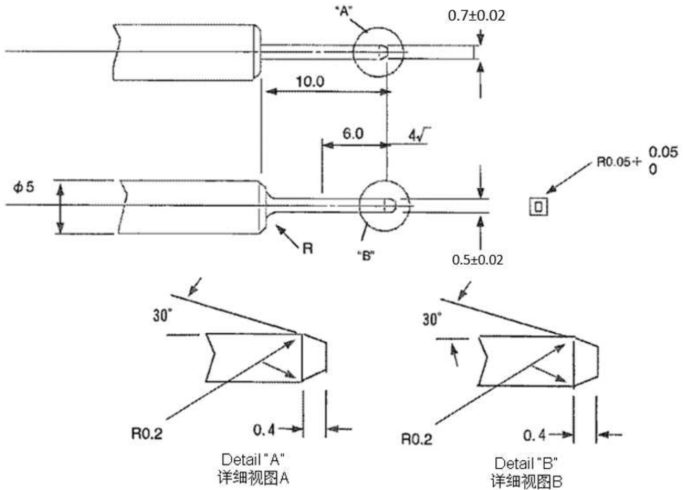
图表 8 端子插拔力测试用量规规格
