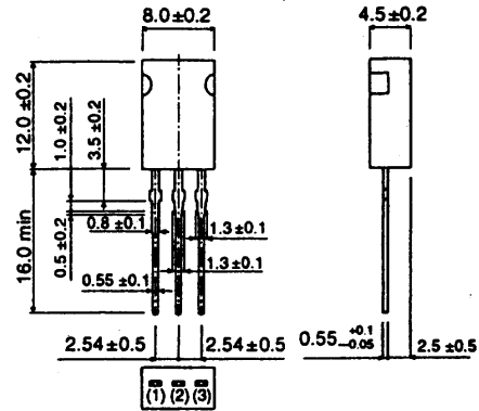
2SD2096 (HRT)
