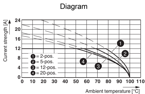
Type: MSTB 2,5/...-ST AU with MSTBA 2,5/...-G AU
