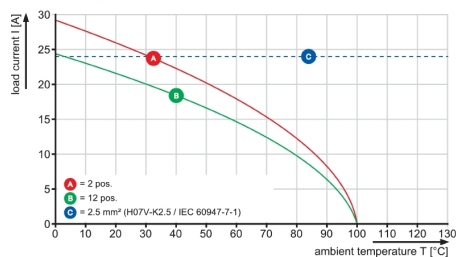
BLF 5.08HC/./180 - SLF 5.08HC/./180
