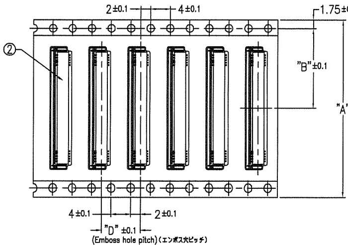
VIEW "A" (N.S.) 矢視 "A" (N.S.)
