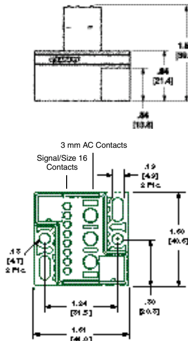
Receptacle 194279-1
