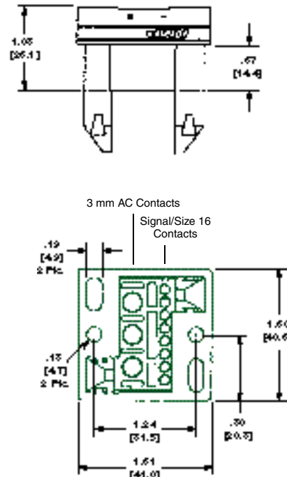
Plug 194278-1
