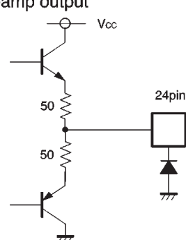
Op-amp output
