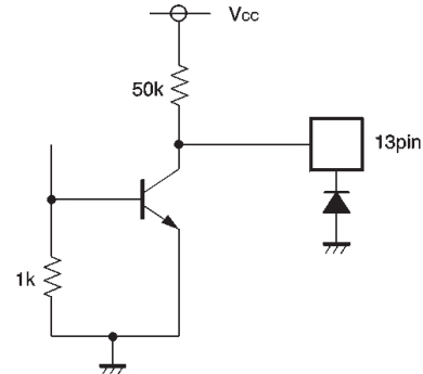
Bias-drop mute
