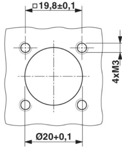
Einbaumaße RF-...N8AWA00, RF-...N8AWB00
