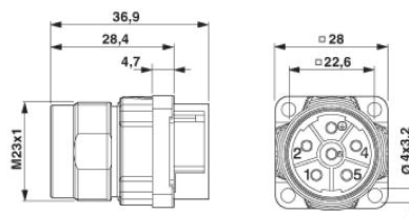
Einbaumaße SF-...P1N8AWK00
