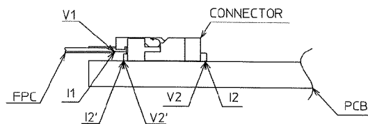
図 1. 接触抵抗測定方法
