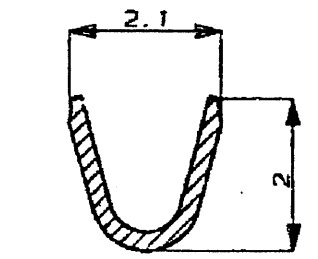
断面 A-A (尺度10-1)
