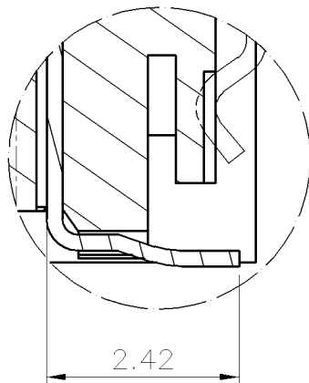
DETAIL A 2:1
