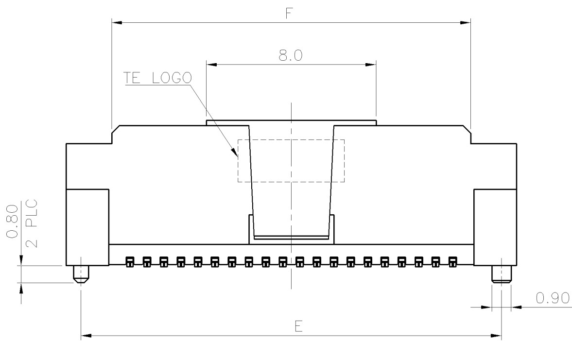
DETAIL A 2:1
