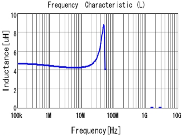
■ 1231AS-H-4R7M L
