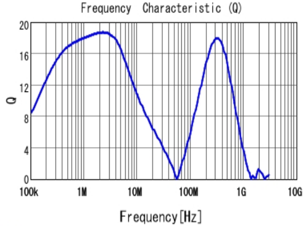
■ 1231AS-H-4R7M Q
