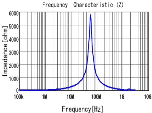
■ 1231AS-H-4R7M |Z|
