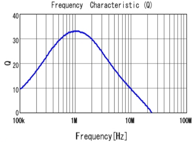
■ 1269AS-H-100N Q
