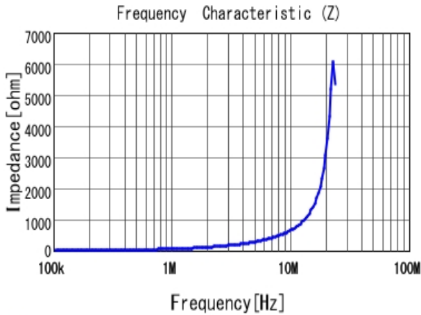
■ 1269AS-H-100N |Z|
