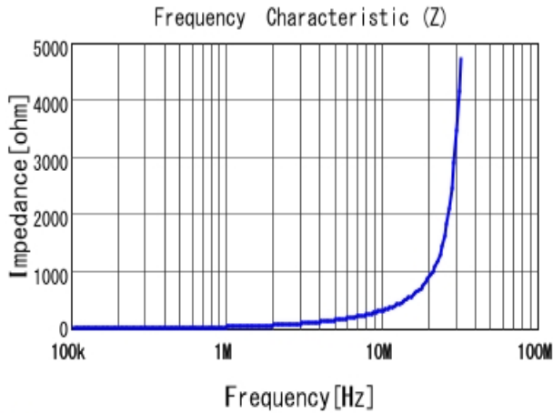
■ 1269AS-H-4R7M |Z|
