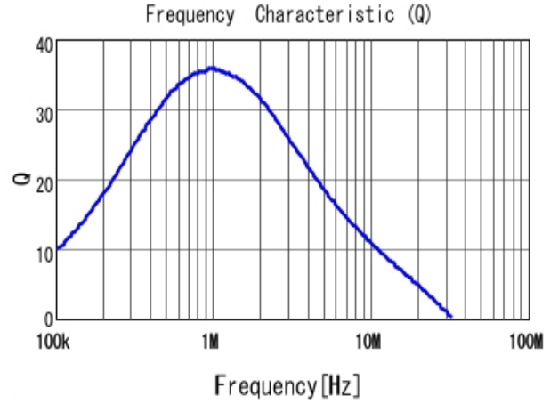
■ 1269AS-H-4R7M Q
