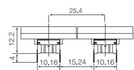
multimec® 3AT + 1M
