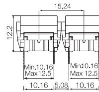
multimec® 3AT + 1B/C + 2A/B
