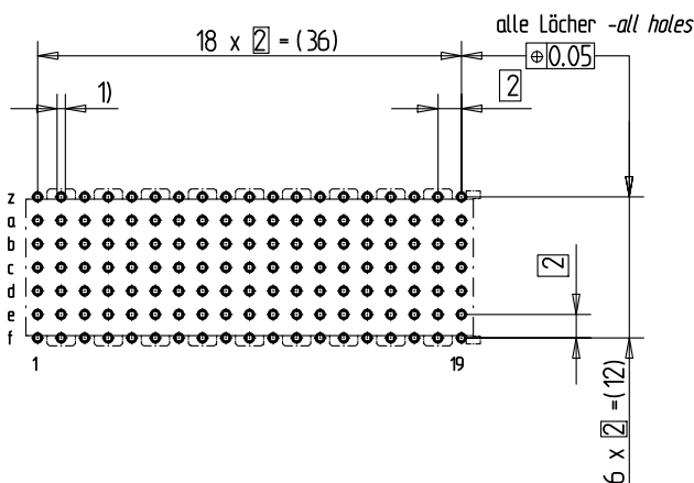
Lochbild für Leiterplatte Board hole pattern (Component mounting side)
