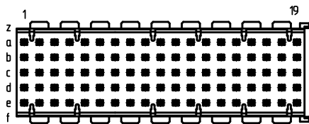
Bestückungsplan - contact layout
