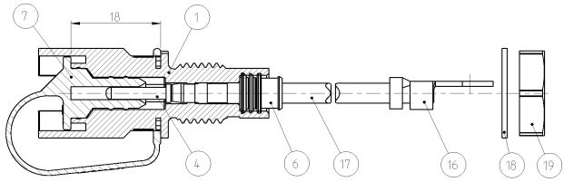
SECTION A-A SCHNITT A-A
