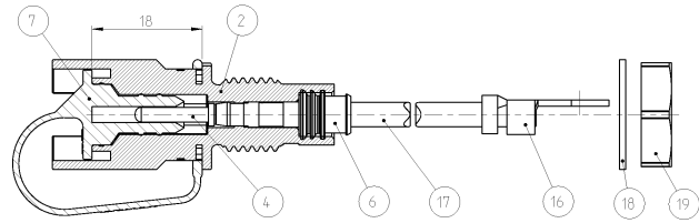
SECTION A-A SCHNITT A-A
