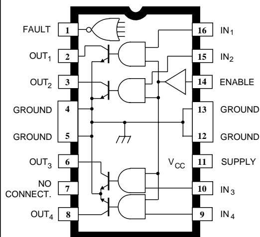
UDx2547B (DIP)
