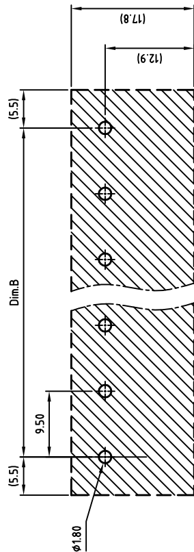
P.C.B Layout
