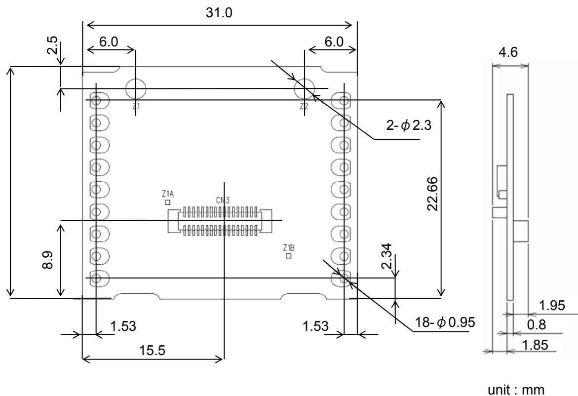
図2 外形寸法図(*)
