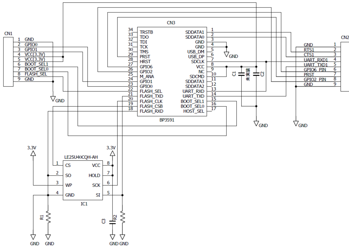
図 4 BP359D 回路図
