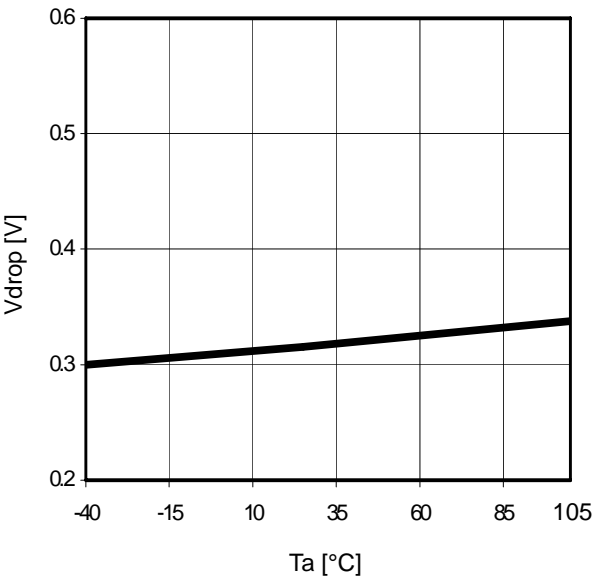
Fig. 33 T_a - V_{drop} ( V_{CC}=6\text{V} , I_o=0.5\text{A} )
