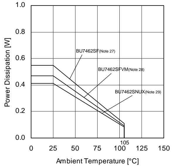
(f) BU7462Sxxx
