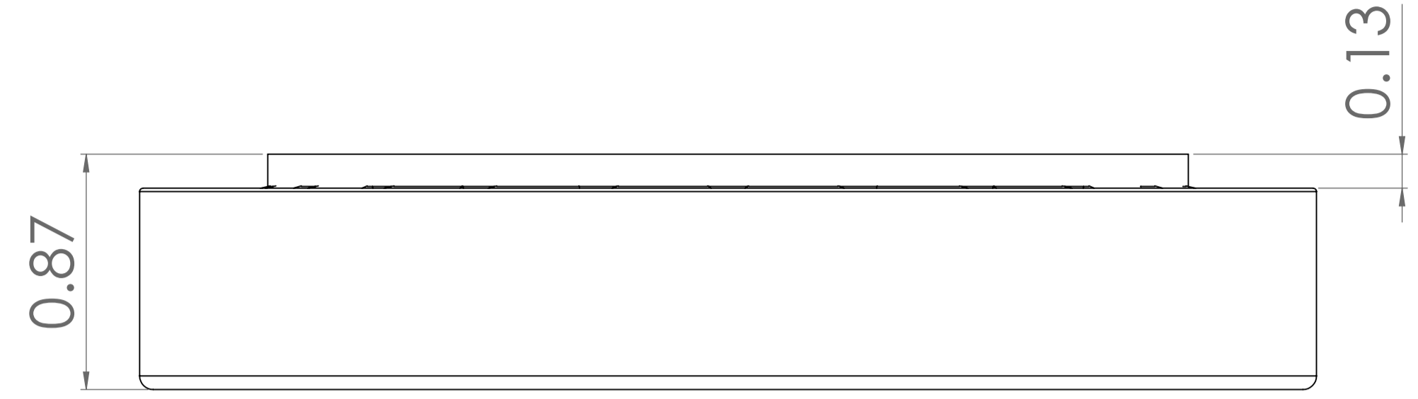
TOP
