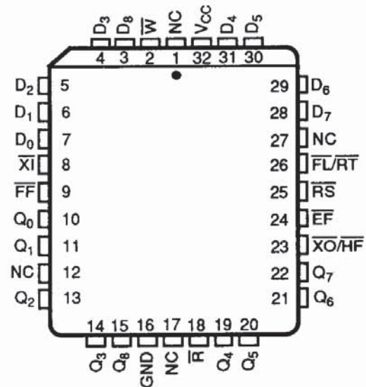
PLCC*
