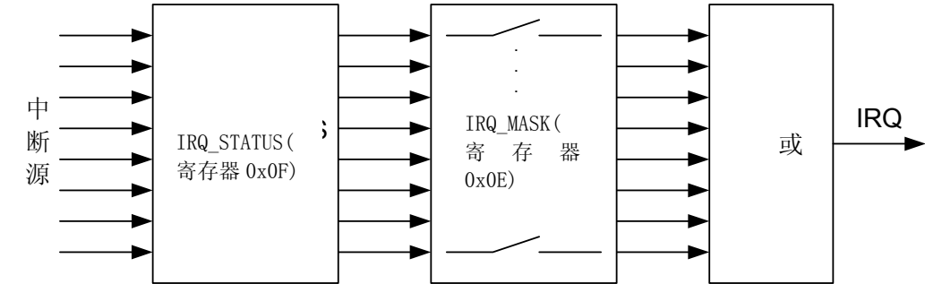
图 4-18 IRQ_MASK_MODE=1
