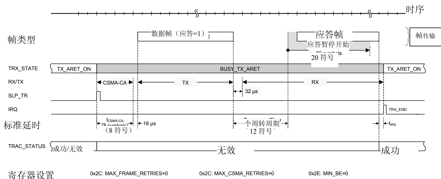
图 5-13 TX_ARET 处理时序示例（无待 ACK 帧待处理数据位设置）
