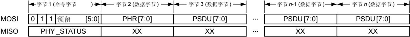
图 4-8 数据包结构-帧写入访问
