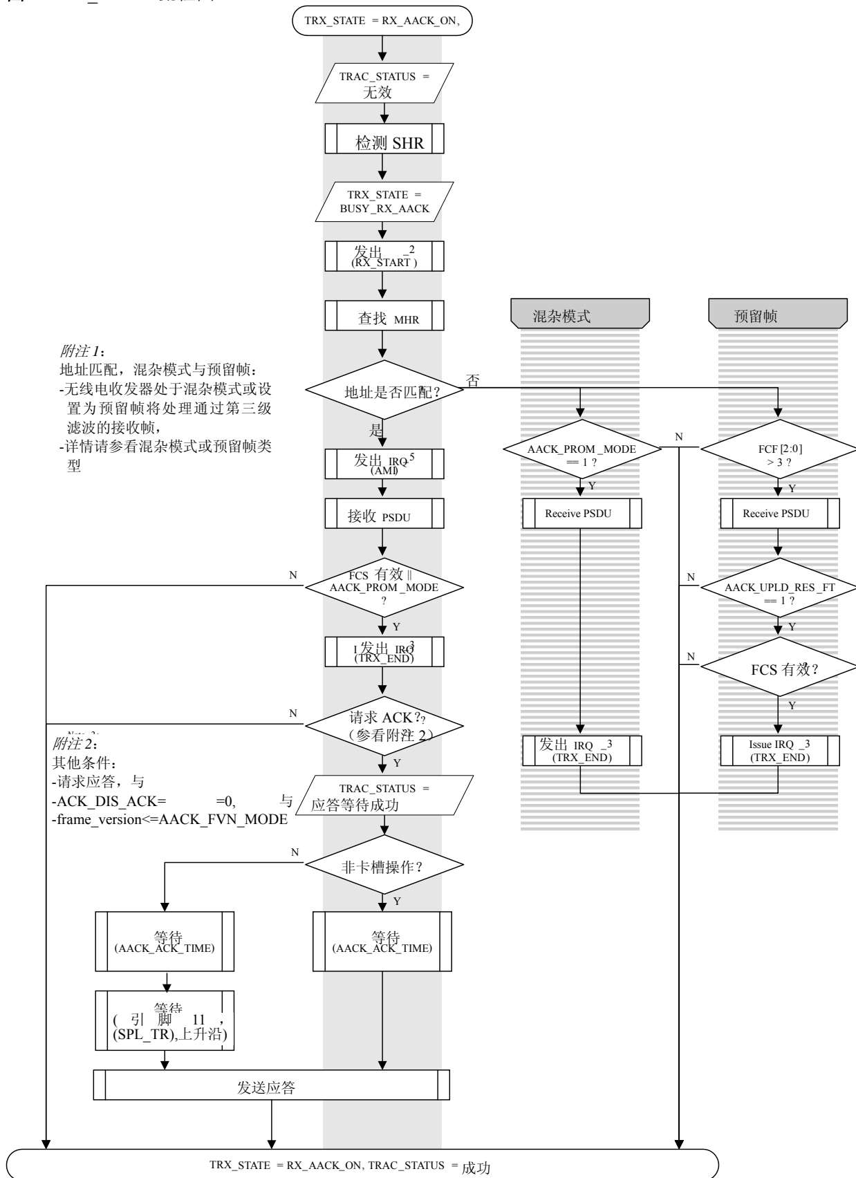
图 5-9 RX_AACK 流程图
