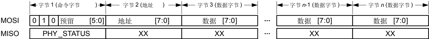
图 4-12 数据包结构-SRAM 写入访问
