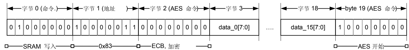
图 9-1. ECB 编程 SPI 时序-加密
