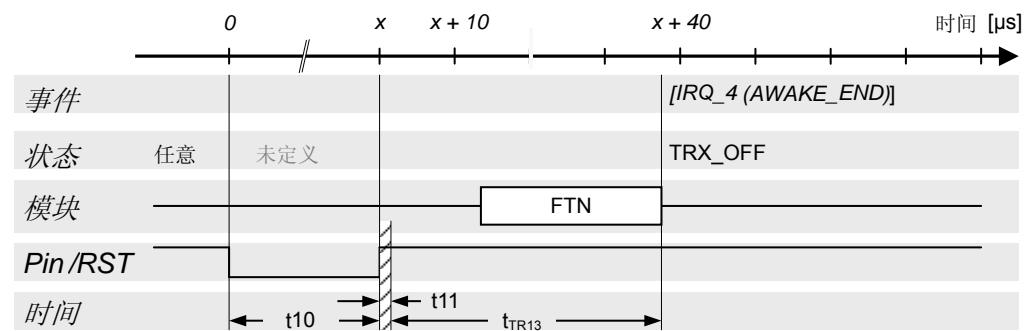
图 5-7 复位程序
