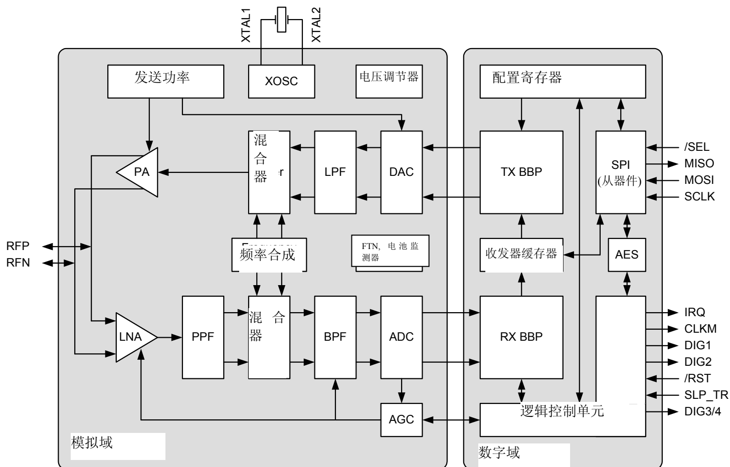
图 1-1 AT86RF212 结构图
