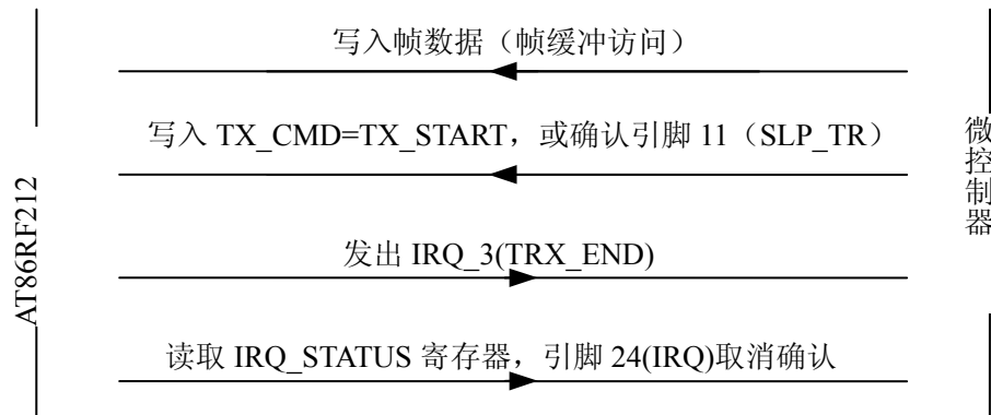
图 8-2 AT86RF212 与微控制器之间的发送处理
