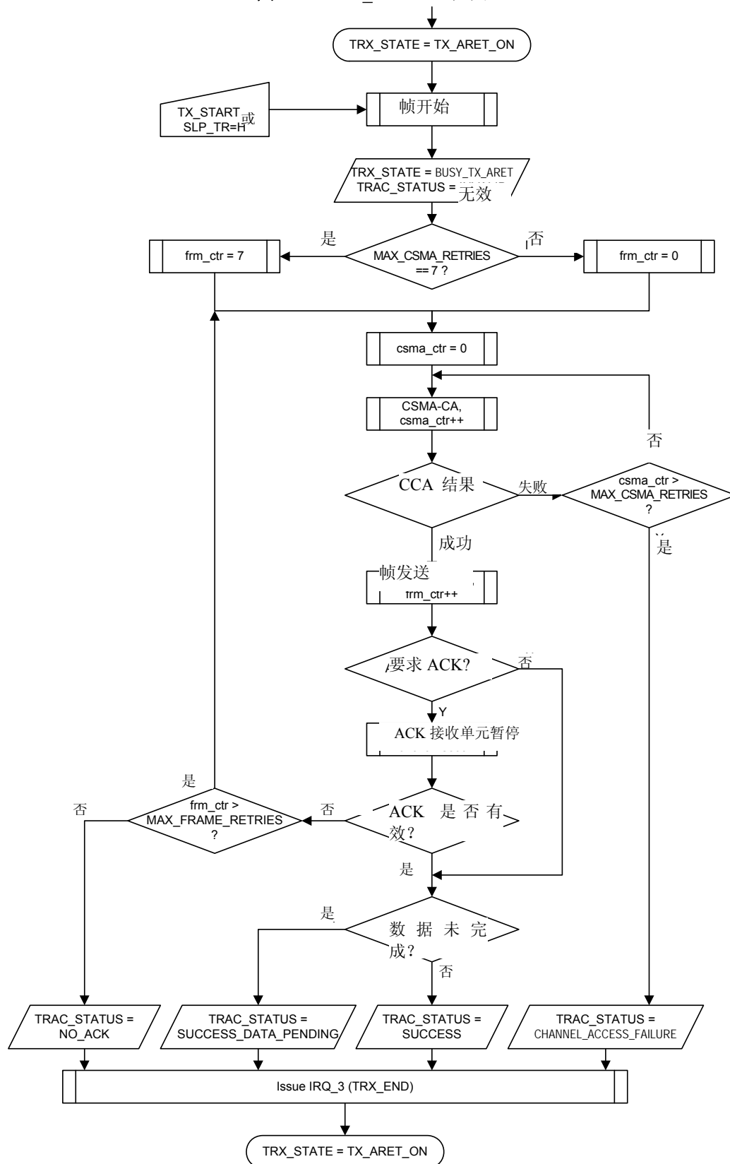
图 5-12 TX_ARET 流程图
