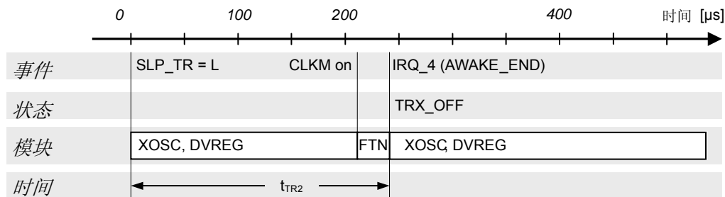
图 5-4 睡眠模式唤醒程序
