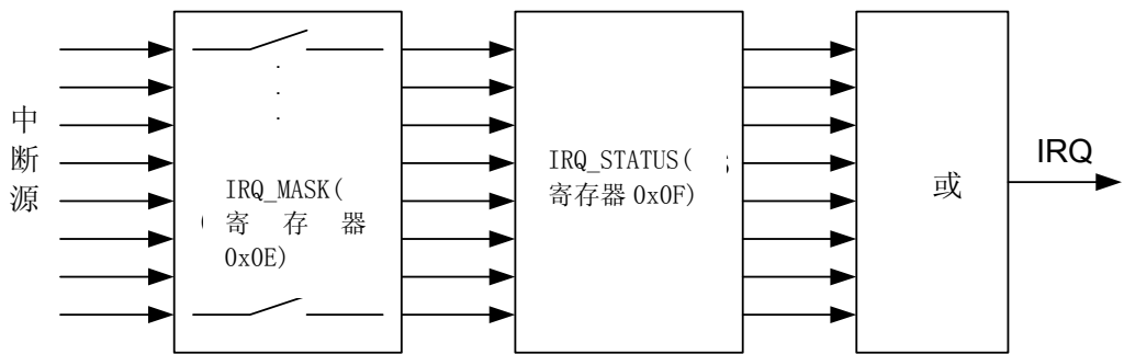
图 4-17 IRQ_MASK_MODE=0
