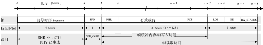
图 7-11. AT86RF212 帧结构
