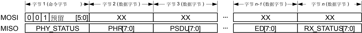
图 4-7 数据包结构-帧读取访问
