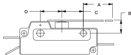
FIG. 7 Lever
