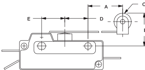
FIG. 3 Lever Roller
